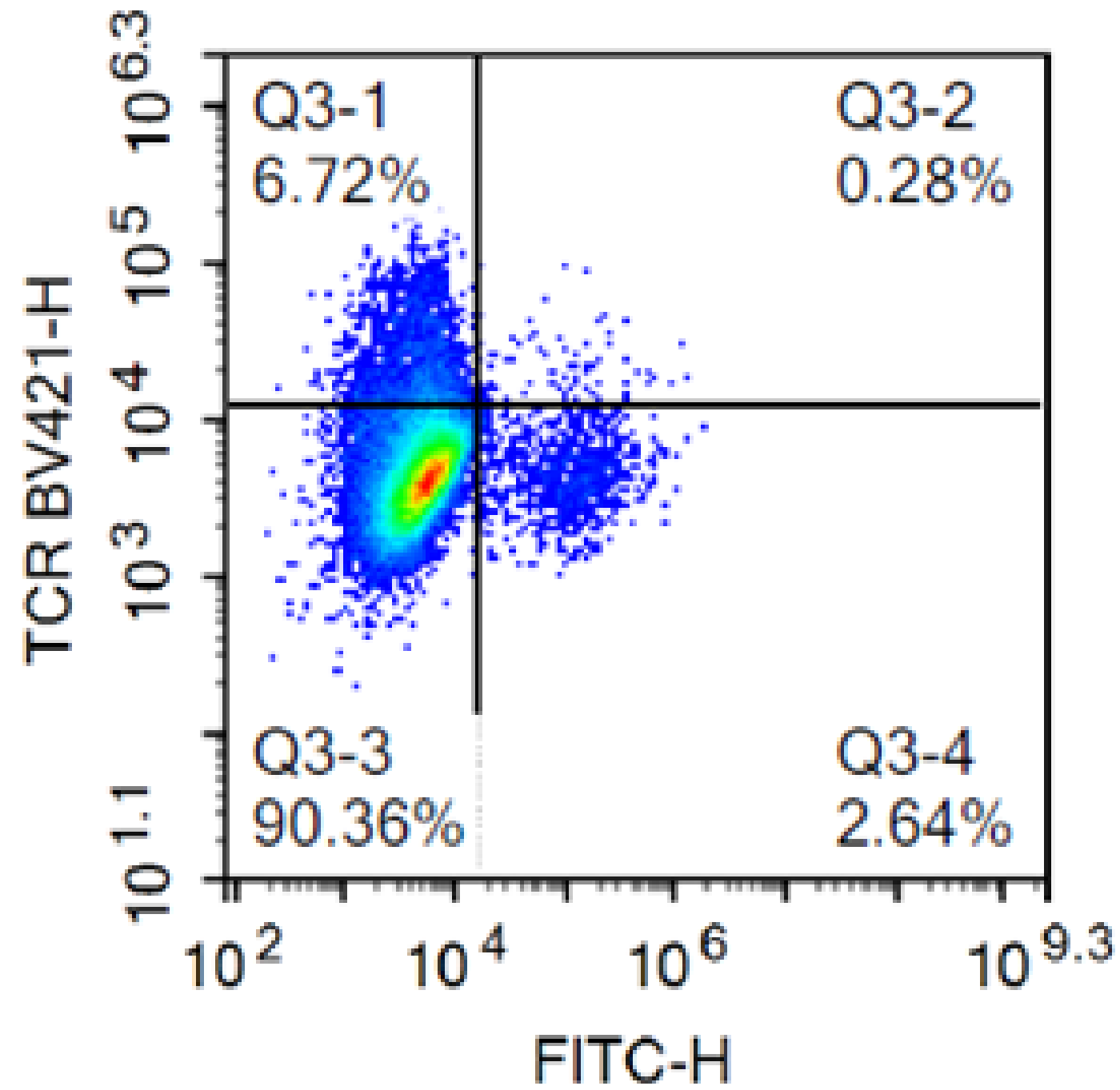
PCR dsDNA
