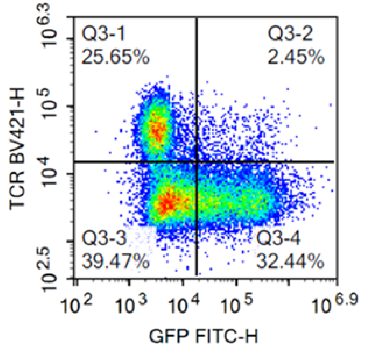
GenWand™ dsDNA
